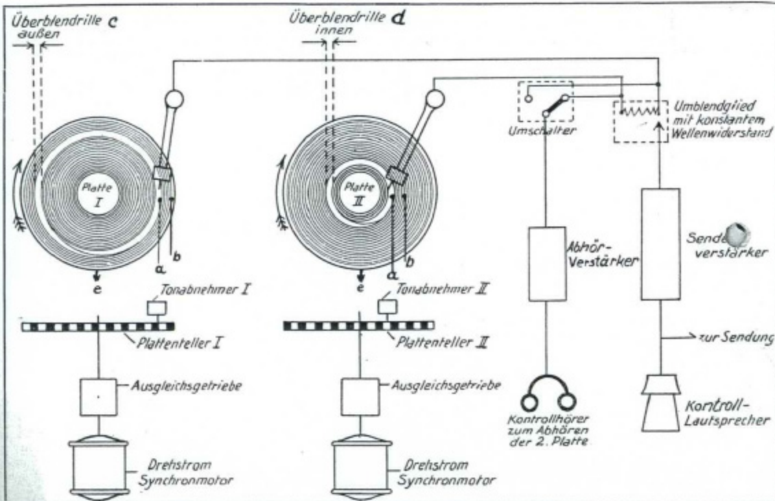
(2) Schema einer vollständigen Schallplatten-Wiedergabeeinrichtung
